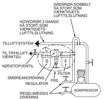
(Dwg. TPD905-2)
